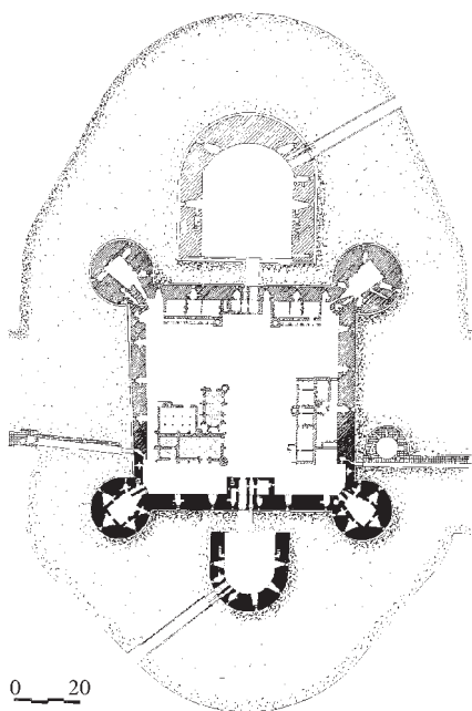
2. KÉP. A DIJONI CITADELLA ALAPRAJZA
