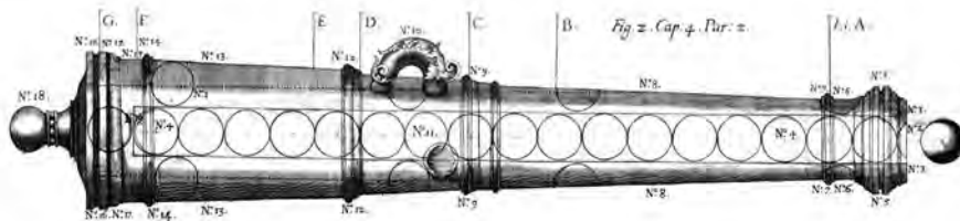
6. KÉP. EGY 16. SZÁZADI BRONZ OSTROMÁGYÚ KERESZTMETSZETI RAJZA. MEGMUTATJA, HOGYAN MÉRETEZTÉK A LÖVEGEKET A GOLYÓ ÁTMÉRŐJE ALAPJÁN
