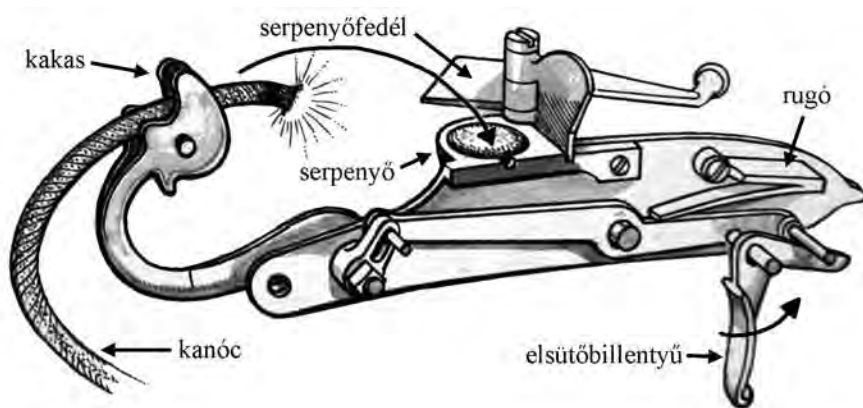
16. KÉP. A KANÓCOS LAKAT
