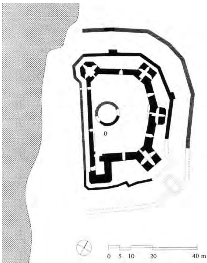
12. KÉP. RÁMA VÁRÁNAK ALAPRAJZA
