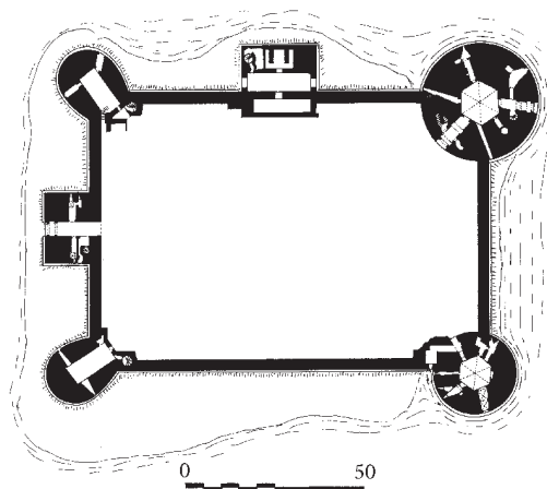
1. KÉP. HAM VÁRÁNAK ALAPRAJZA
