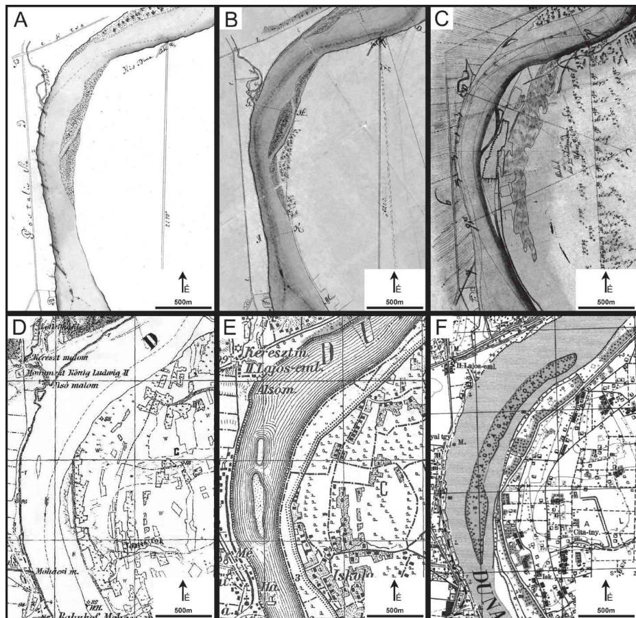
2. ÁBRA. A CSELE-PATAK TORKOLATA ALATTI DUNA-SZAKASZ ZÁTONYOKKAL, SZIGETEKKEL ÉS A KELETI PART MENTÉN ÖVZÁTONNYAL. JÓL MEGFIGYELHETŐ A DUNA MEDRÉNEK SZÉLESEDÉSE, ILLETVE A NYUGATI (JOBB) PART ELHORDÁSA (AZ ÚT ÉS A CSELE-TORKOLAT PUSZTULÁSA)
